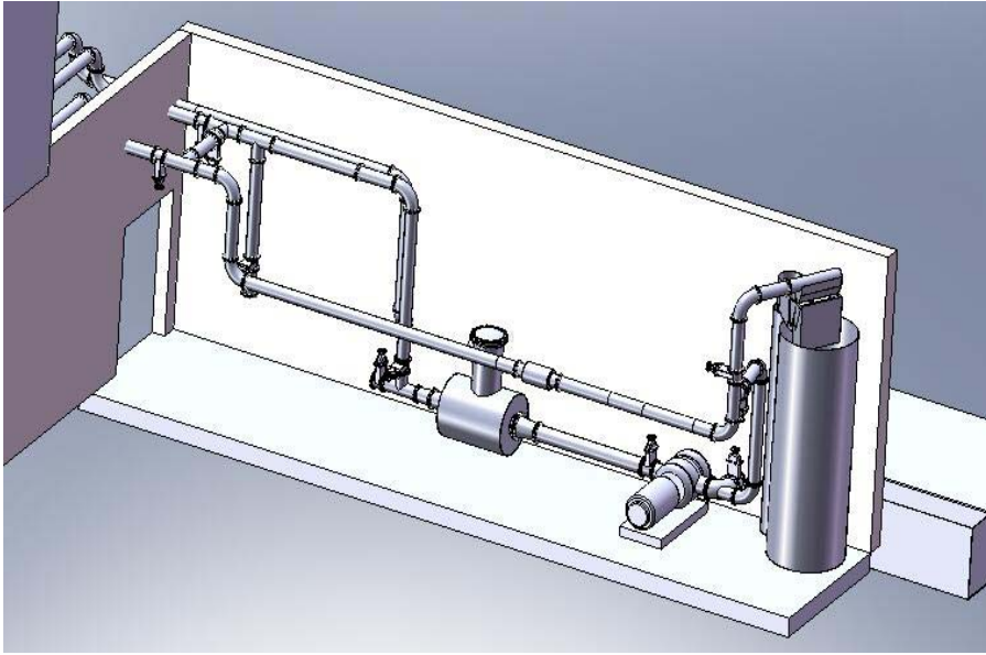
Слика 2. Први део инсталације смештен у подрумским просторијама лабораторије
